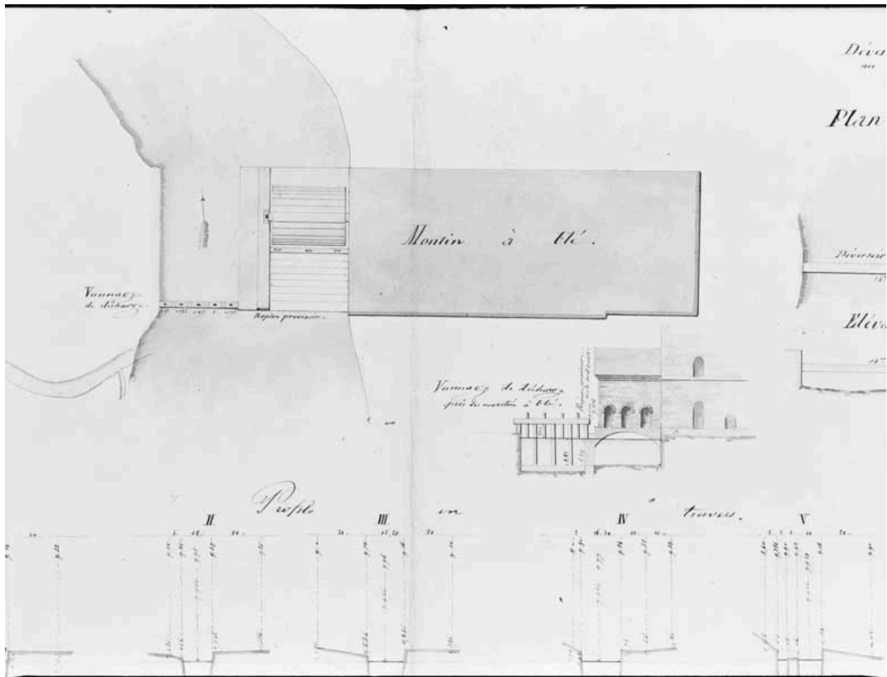
Usine de M. Chauvel. Plan général, plan de détail, projets en long et en travers.- Plan de détail, 1/200e, par Sallebert, ingénieur ordinaire, 14 avril 1857. (AD Calvados. S 12805b).
