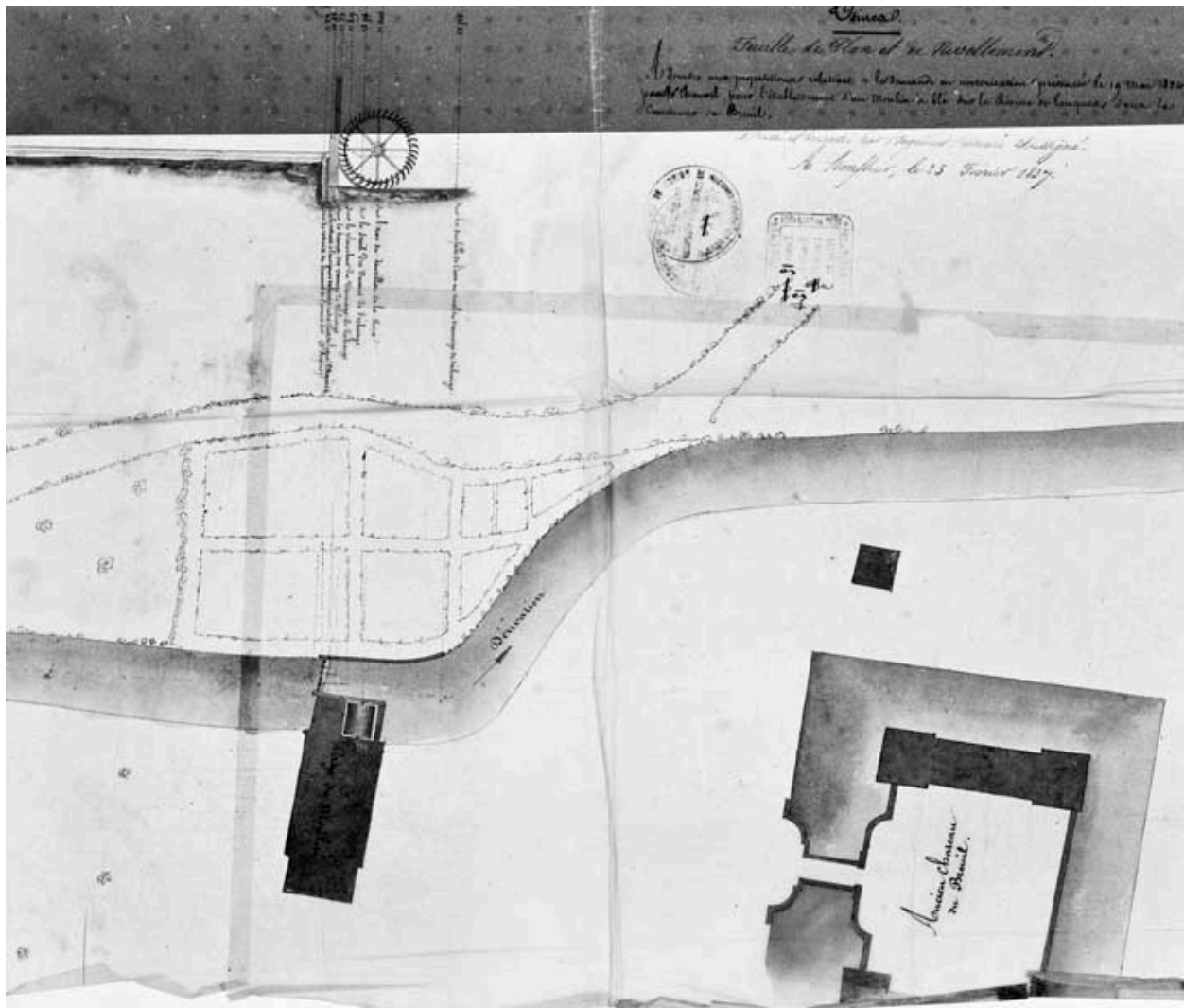
Feuille de plan et nivellement à joindre aux propositions relatives en autorisation, présentées le 19 mars 1834 par M. Chauvel pour l'établissement d'un moulin à blé sur la rivière de Touques dans la commune du Breuil.- Plan, 25 février 1837. (AD Calvados. S 12805b).
