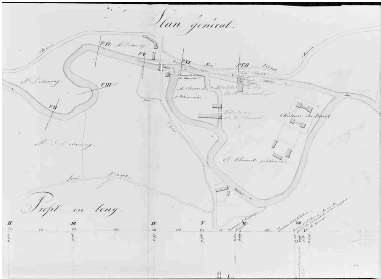
Usine de M. Chauvel. Plan général, plan de détail, projets en long et en travers.- Plan d'ensemble, 1/2500e, par Sallebert, ingénieur ordinaire, 14 avril 1857. (AD Calvados. S 12805b).
